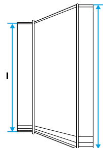
Schéma d'encombrement Réduction Oblongue Tangentielle sur Plat
