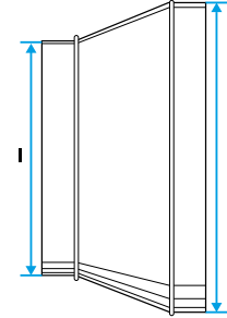
Schéma d'encombrement Réduction Oblongue Tangentielle sur Plat
