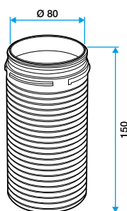
Rallonge circulaire Ø80 mm
