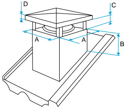
Schéma d'encombrement Sortie de Toit Esthétique
