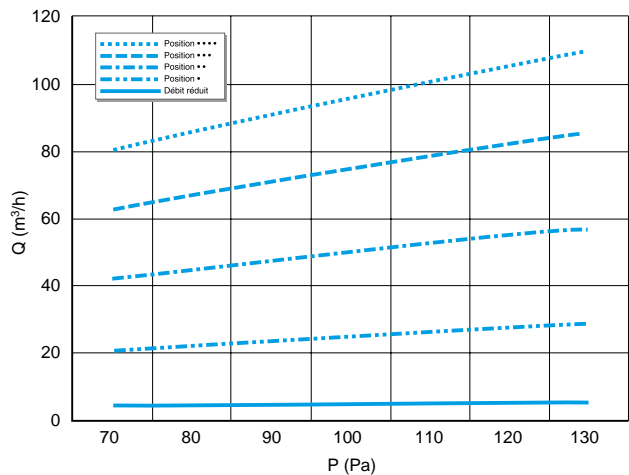
Courbe aéroulique TDA
