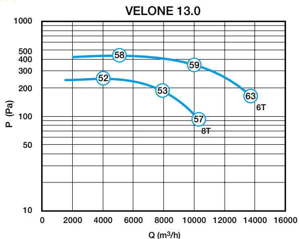
Caractéristiques aérauliques et acoustiques VELONE 13 - 8T 1.1 kW
