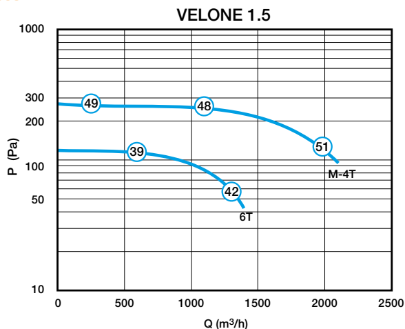
Caractéristiques aérauliques et acoustiques VELONE 1.5M 0.24 KW
