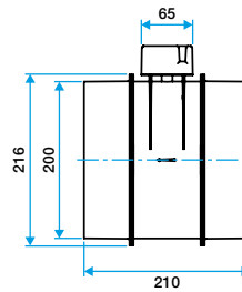
Dimensions RMA D200
